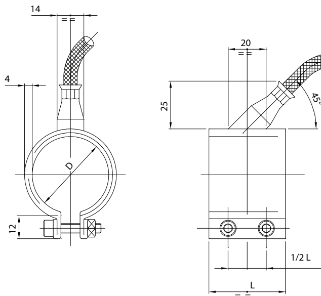
Standard con uscita a 45° assiale ( 30° assiale opzionale ) Cavo bipolare flessibile + terra, lung. 1000 mm
