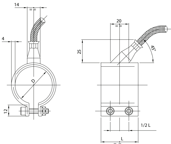
Standard con uscita a 45° assiale Cavo bipolare flessibile + terra, lung. 1000 mm
