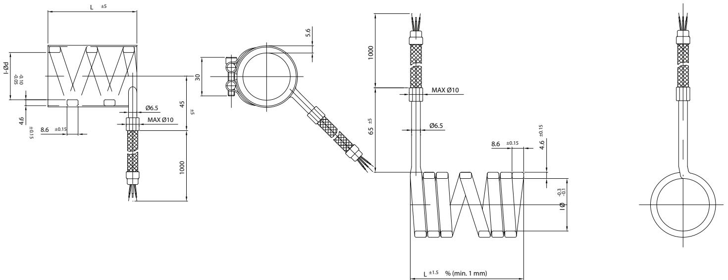
Modello tangenziale con uscita a 45°
