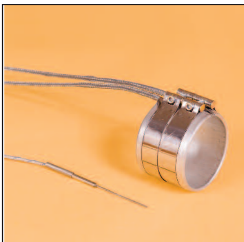
Esempio Z.15 con termocoppia esterna da inserire
