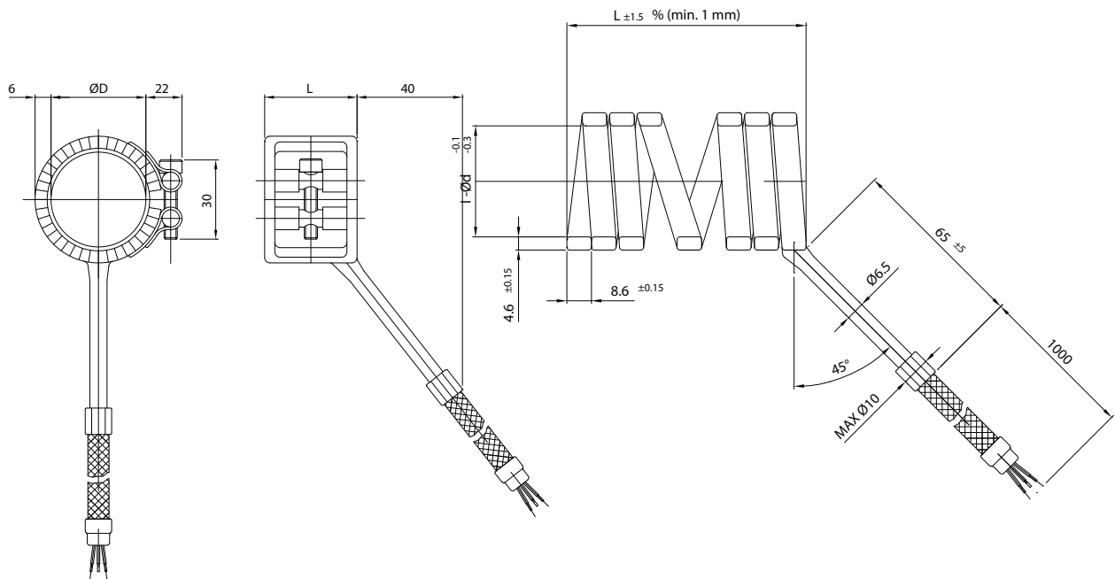
Standard con uscita a 45° assiale con fascetta di chiusura
