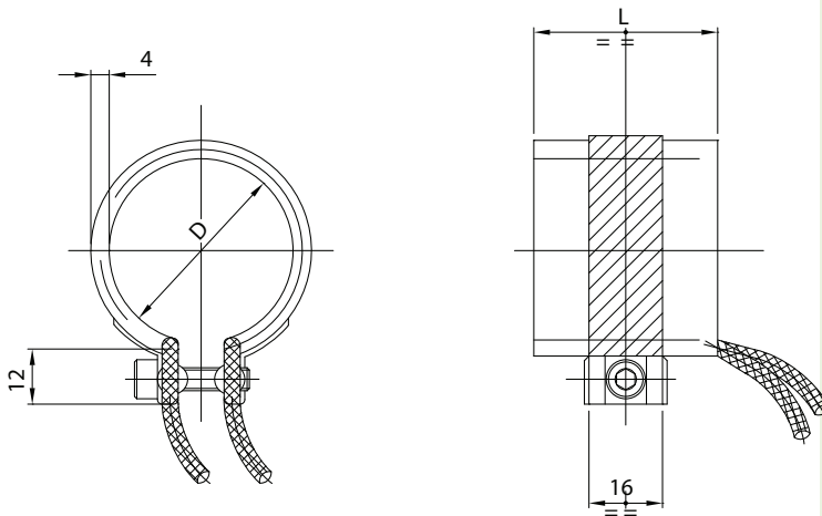
Nr. 1 fascetta fino a L 35 mm Nr. 2 fascette da L 36 mm a L 60mm
