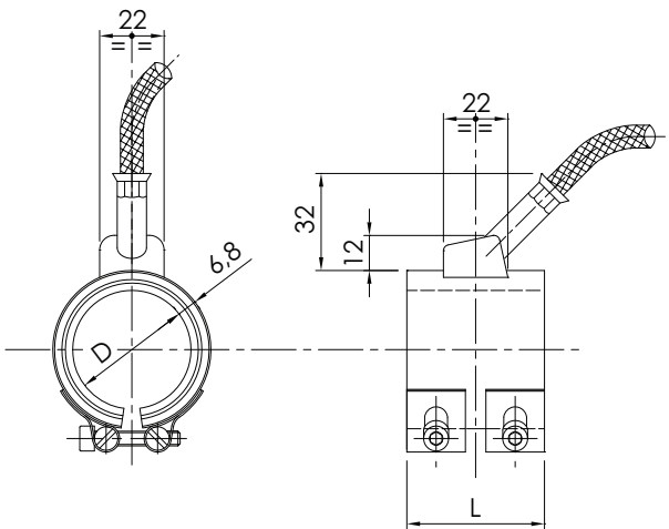
Standard con uscita a 45° assiale ( 30° assiale opzionale )
