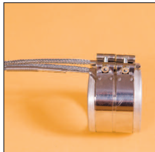
Esempio: Z.15 con termocoppia esterna installata nella resistenza
