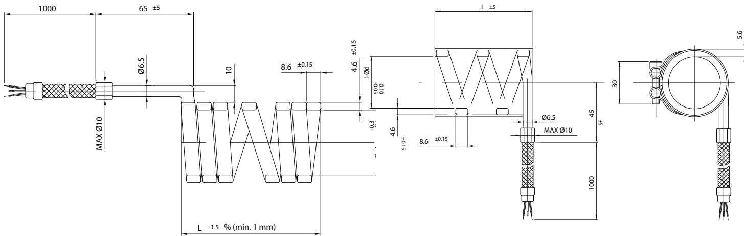
Modello assiale con uscita a 0°
