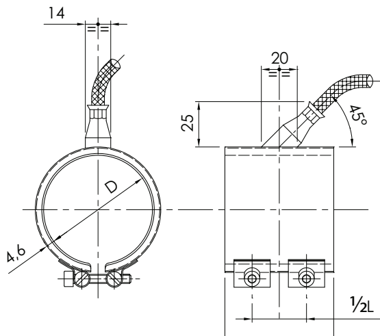
Standard con uscita a 45° assiale ( 30° assiale opzionale )
